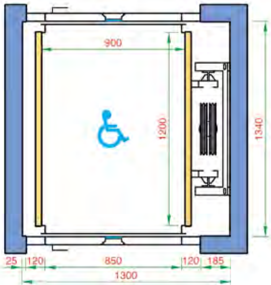
MLT MODELLO 5 - 2 ACCESSI L.
