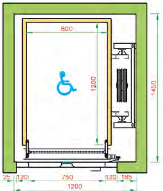
MLTP MODELLO 3 - 1 ACCESSO L. - SOFF.
