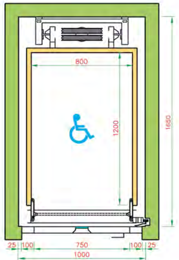
MLTP MODELLO 3 - 1 ACCESSO P. - SOFF.
