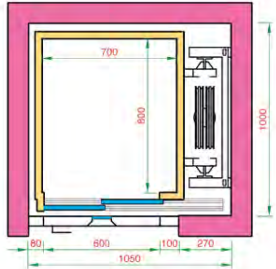
MLTP MODELLO 1 - 1 ACCESSO L. - 2 A
