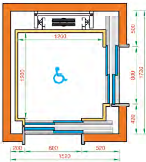
MLTP MODELLO 10 - 2 ACCESSI 90° - 2 A
