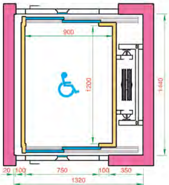
MLTP MODELLO 5 - 2 ACCESSI L. - 2 A
