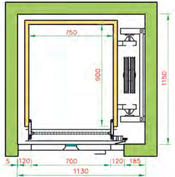
MLTP MODELLO 2 - 1 ACCESSO L. - SOFF.
