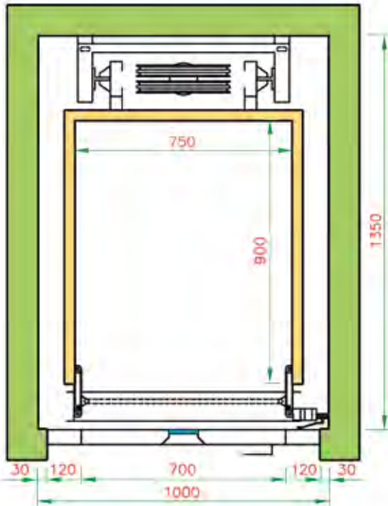
MLTP MODELLO 3 - 1 ACCESSO L. - SOFF.
