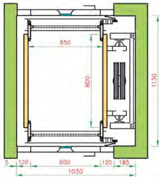
MLTP MODELLO 1 - 2 ACCESSI L. - SOFF.
